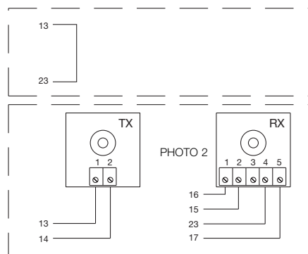
Fig 3C Connexion photo-test avec seulement la photocellule Photo2
