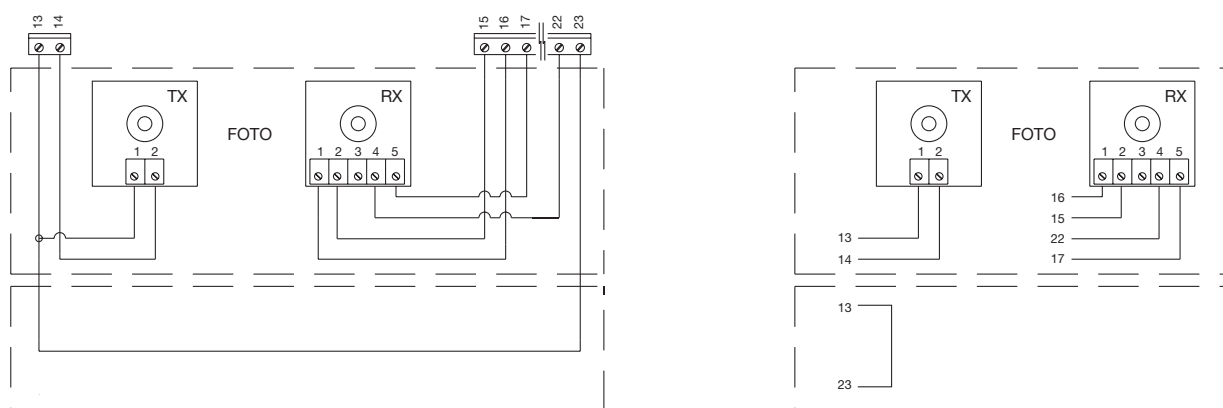
Fig 3B Collegamento fototest con la sola fotocellula Foto
