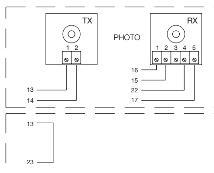
Fig 3B Connexion photo-test avec seulement la photocellule Photo
