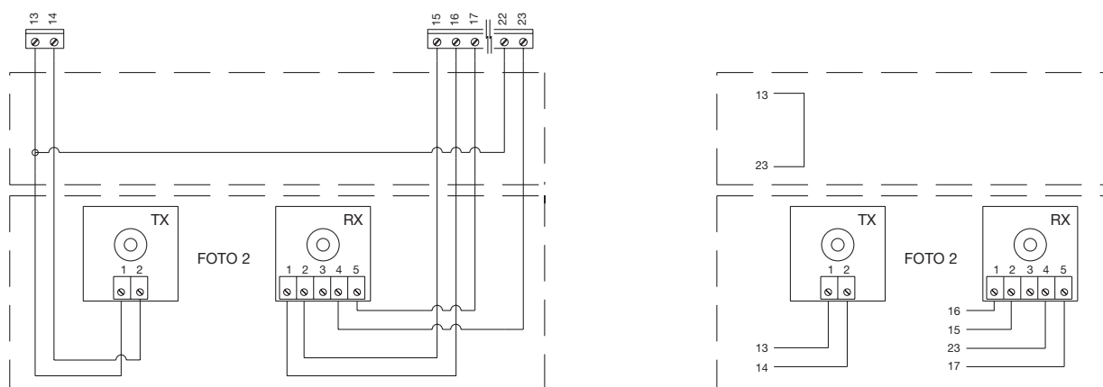
Fig 3C Collegamento fototest con la sola fotocellula Foto2
