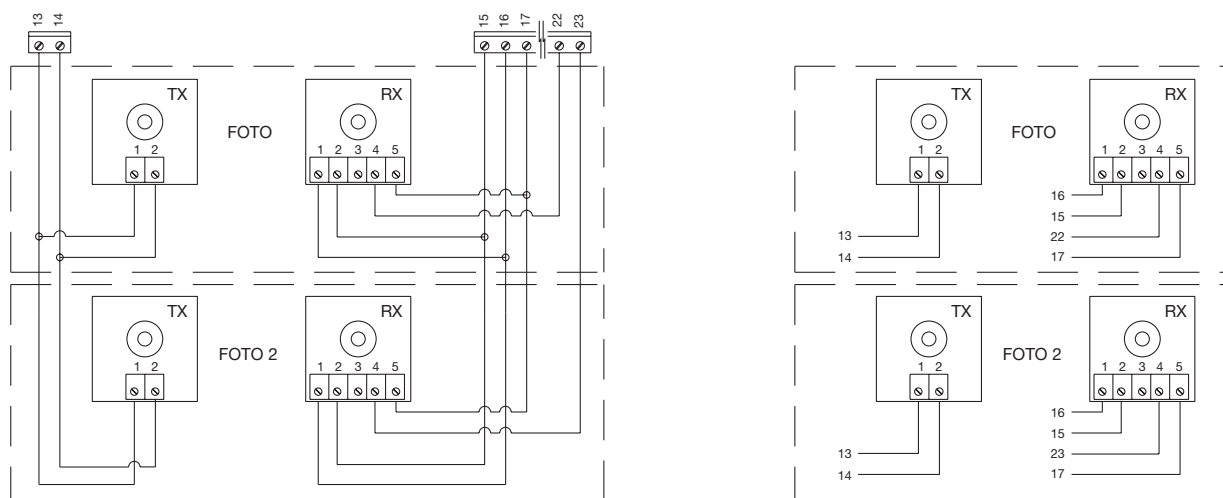
Fig 3A Collegamento fototest con le fotocellule Foto e Foto2
